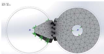
「はすば歯車対」をかみ合わせた場合のFEMによる応力解析モデル
